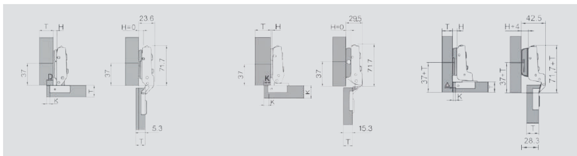
775D(40) H=19+K-D
