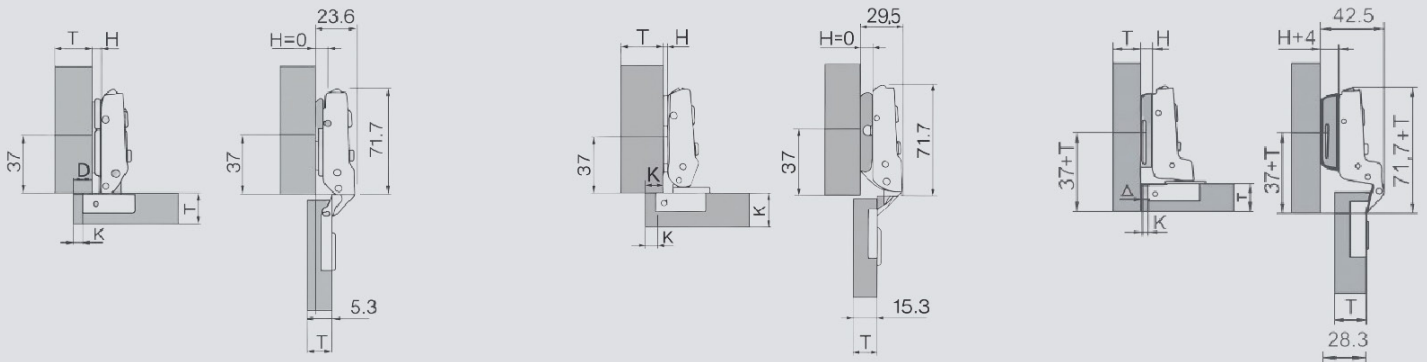
775D(40) H=19+K-D
