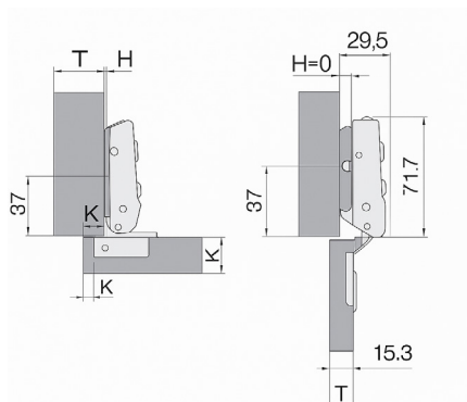
776D(40) H=9+K-D
