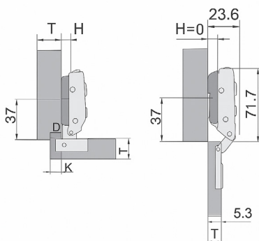
775D(40) H=19+K-D
